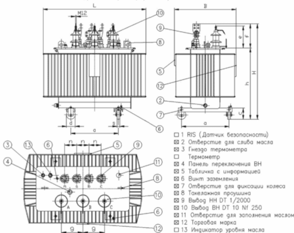
Чертеж трансформатора ТОНн
